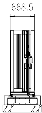
A-A矢视图
