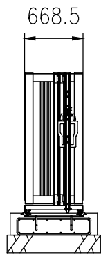
A-A矢视图
