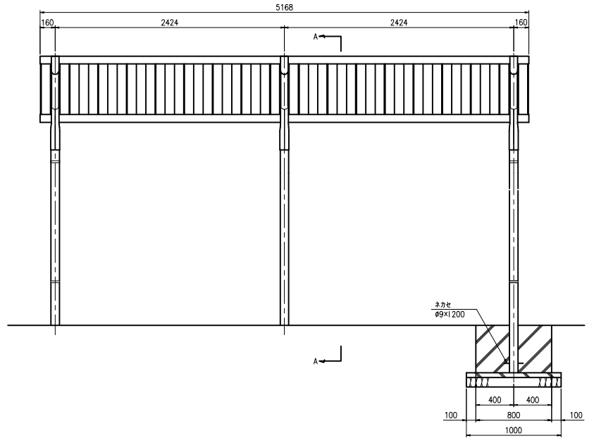
正面図 (S=1:20)
