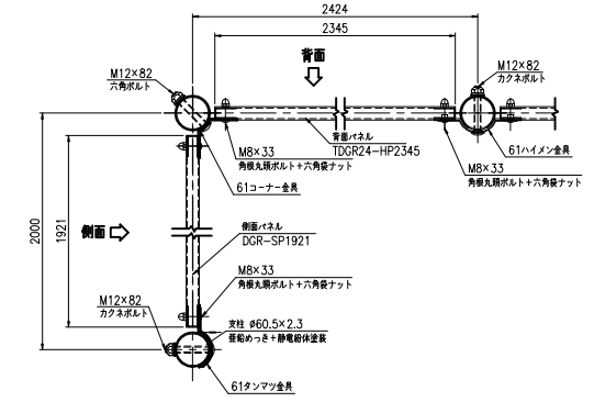
パネル取付詳細図 (S=1:5)
