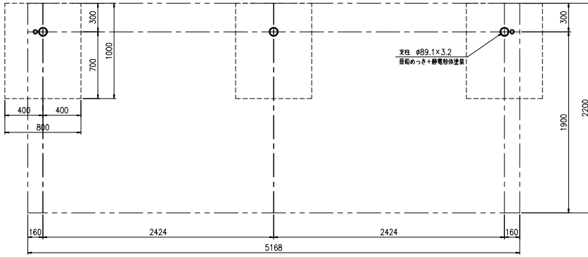
平面図 (S=1:20)
