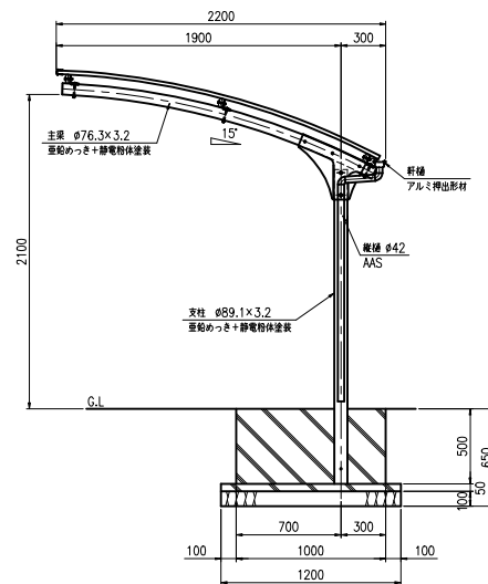
側面図 (S=1:20)
