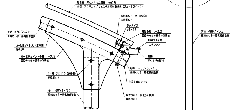
B部詳細図 (S=1:5)
