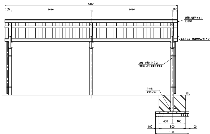
正面図 (S=1:20)
