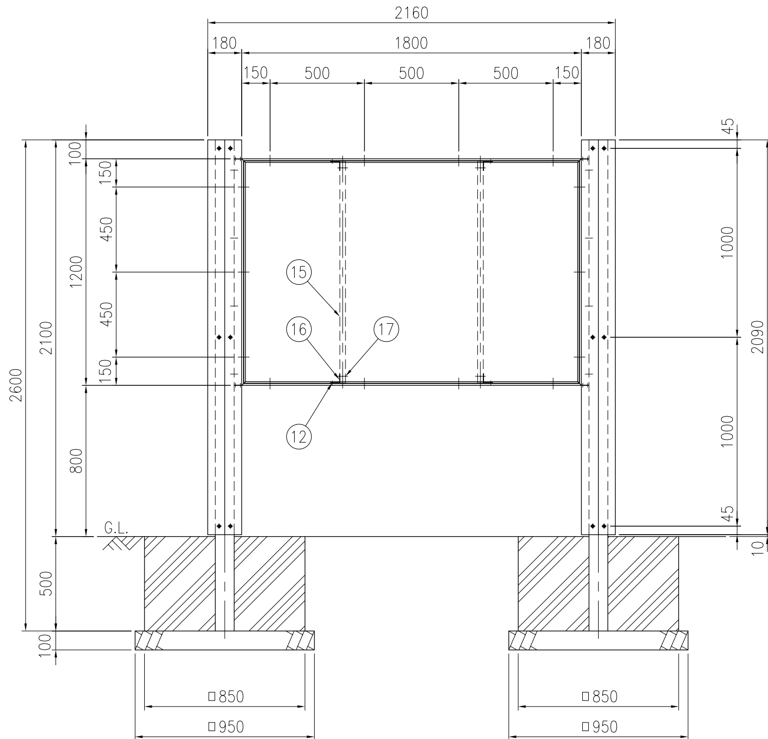
設置図 S=1/20
